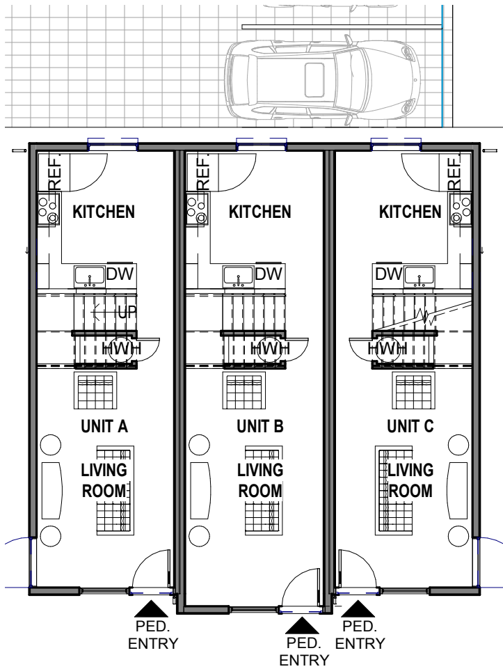
1 LEVEL 1 PLAN #1 :
