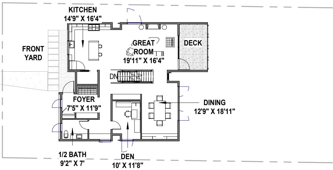
2 LEVEL 1 PLAN :
