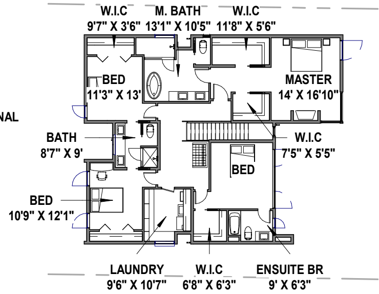
3 LEVEL 2 PLAN :
